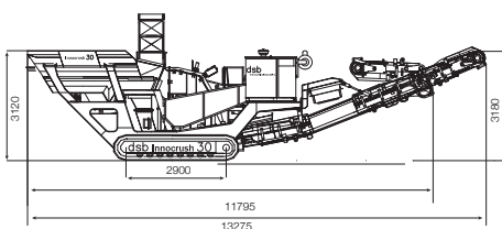
Side view IC 30
